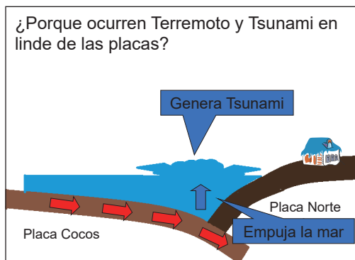
図5 地震・津波が生じるメカニズムの説明に用いた模式図 (中野作成)
