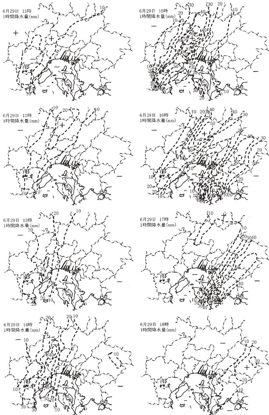
図14 広島県西部における1999年6月29日11時から18時までの時間降水量の分布
