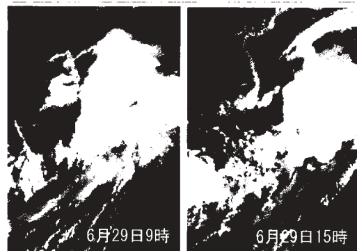
図1 1999年6月29日9時の地上天気図((財)日本気象協会, 1999)、9時と15時の気象衛星「ひまわり」の赤外画像(高知大学気象情報頁, 1999)
