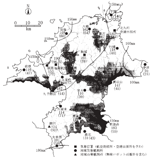
図3 福岡県における1999年6月29日の日降水量の分布
