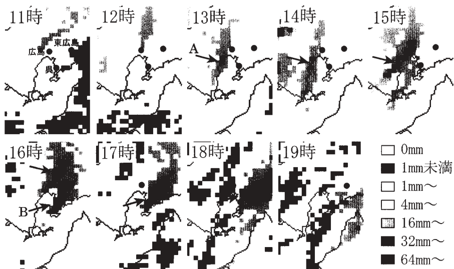
図8 6月29日11時から19時までの1時間毎のレーダーアメダス合成図((財)気象業務支援センター, 1999b に加筆) 図の●は、広島(地方気象台)、呉(測候所)、東広島(地域気象観測所)の位置を示す
