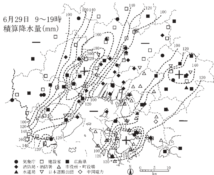
図13 広島県西部における1999年6月29日の9時から19時までの積算降水量の分布図
