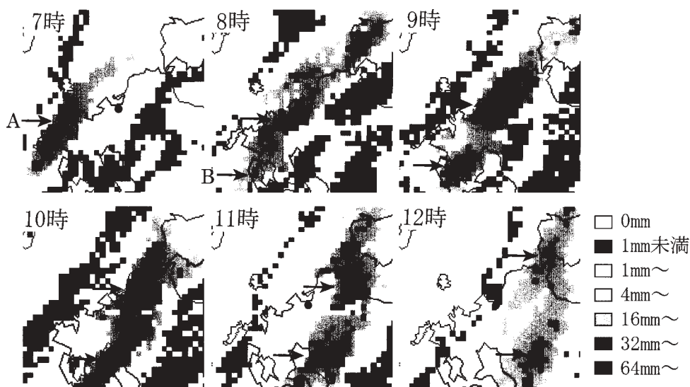
図2 6月29日7時から12時までの1時間毎のレーダーアメダス合成図((財)気象業務支援センター, 1999b に加筆) 中央の●は、福岡管区気象台の位置を示す
