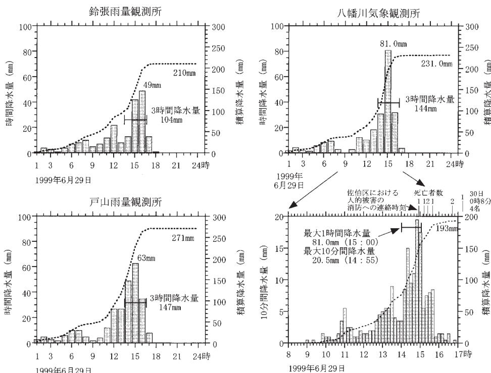
図12 鈴張（雨量観測所）、戸山（雨量観測所）、八幡川橋（気象観測所）における1999年6月29日の1時間・10分間降水量およびその積算値の推移
