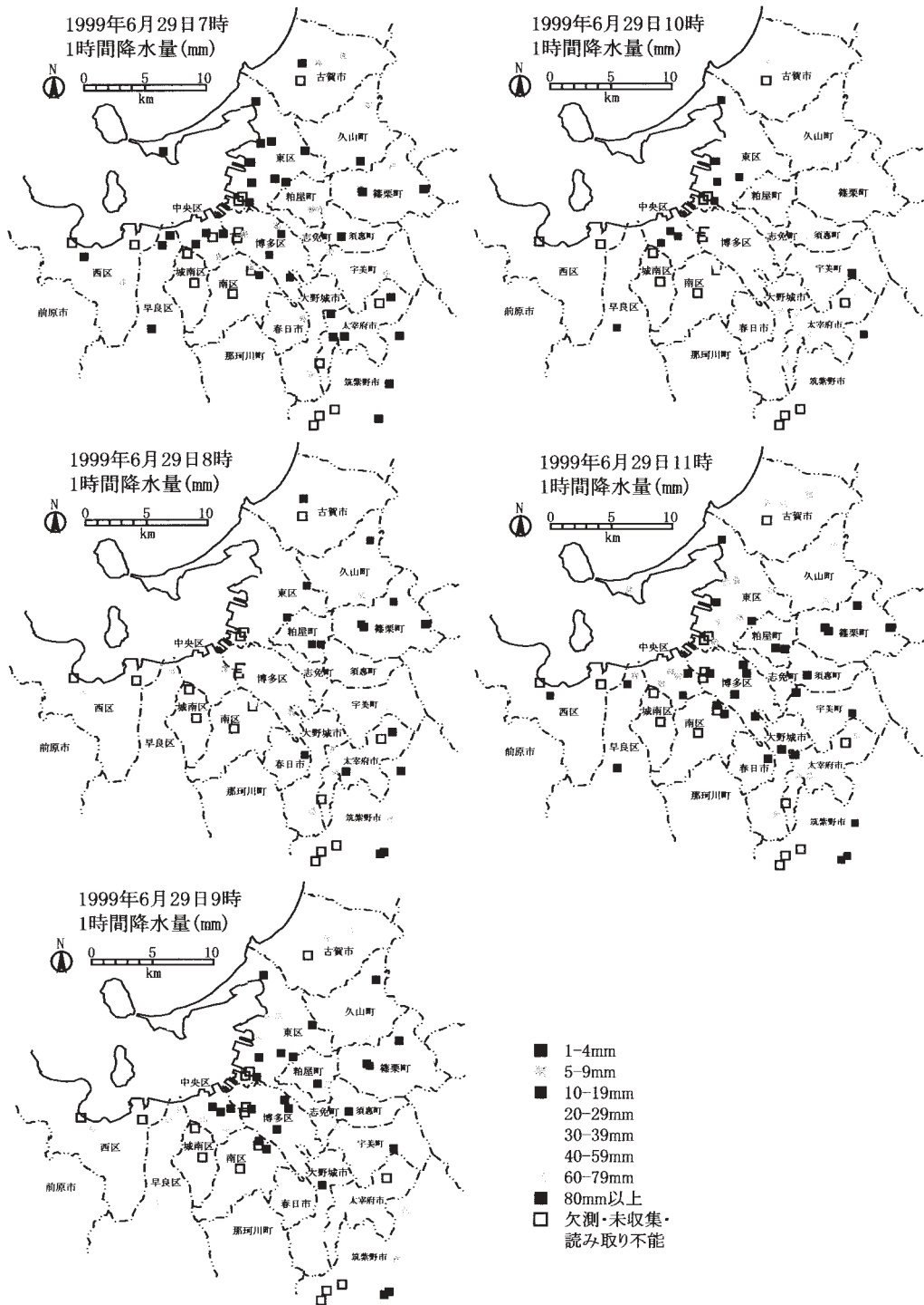
図7 福岡市およびその周辺地域における1999年6月29日7時から11時までの時間降水量の分布
