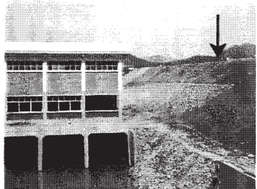
写真5 矢印付近が堤防決壊部。左がポンプ場。この堤防の反対側が黄江遊水部。手前が氾濫域。
