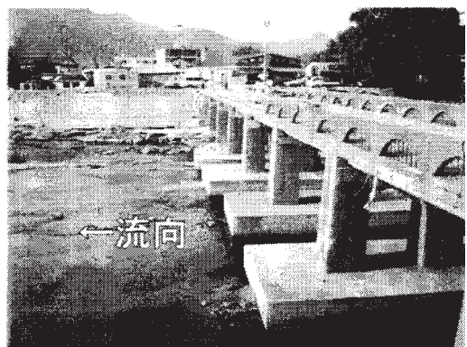
写真 8 草江にかかる黄澗橋。下流側(左側)コンクリート欄干が流失している。
