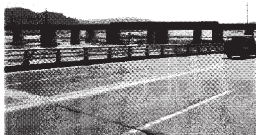
写真 6 甘川の落橋箇所。桁の形が違って2桁が落橋した。
