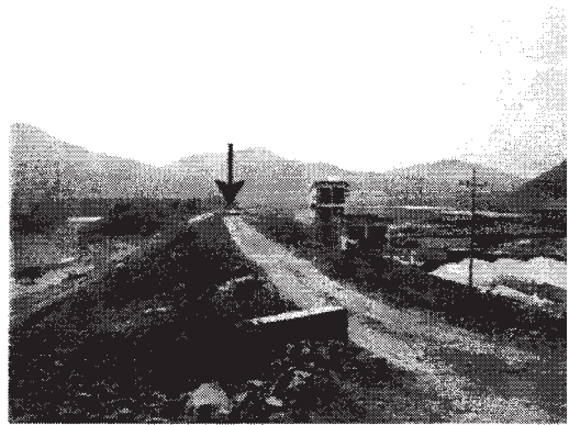
写真4 新反川左岸の決壊部(矢印)。中央に見える建物がポンプ場。堤体は応急工事で復旧されている。
