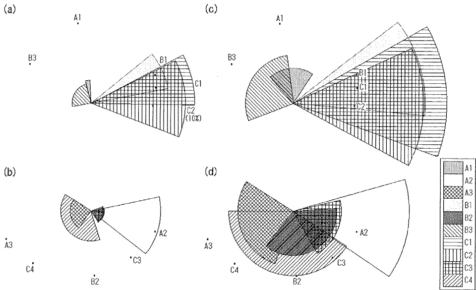
図4 2002年5月～2003年4月の山麓の各観測局における高濃度SO 2 事象の発生割合と八丈島925 hPa風との関係。1年間の高層風・SO 2 データが共に得られた時間数に占める割合を面積で表す。(a)北半部の局での1 ppm以上の割合, (b)南半部の局での1 ppm以上の割合, (c)北半部の局での0.1 ppm以上の割合, (d)南半部の局での0.1 ppm以上の割合
