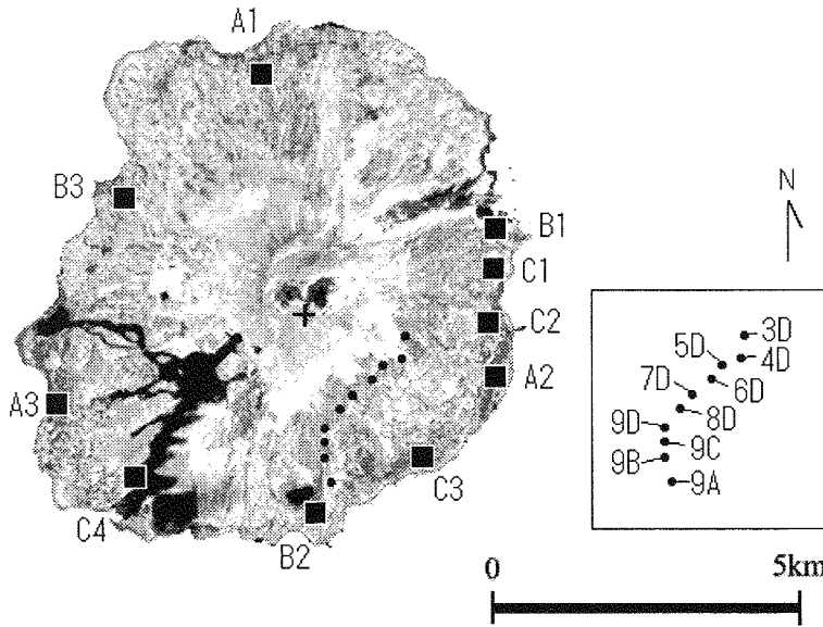
図2 三宅島山麓(■)と山腹(●)の火山ガス観測局の位置(山麓の局名は表1に示す。山腹の局名は四角の枠の中に示す)
