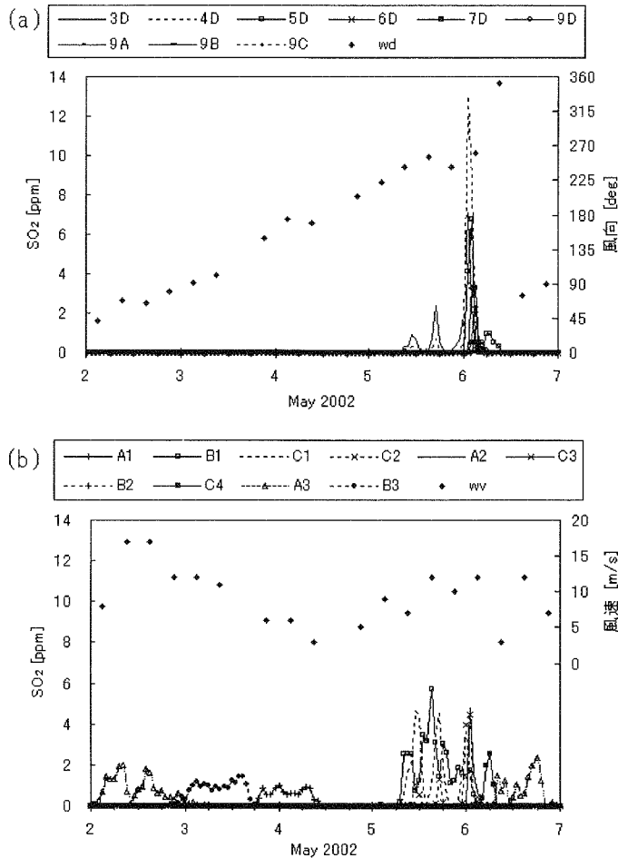
図9 2002年5月2～6日のSO 2 濃度の時系列変化と八丈島925 hPa風 (a) 山腹局, (b) 山麓局
