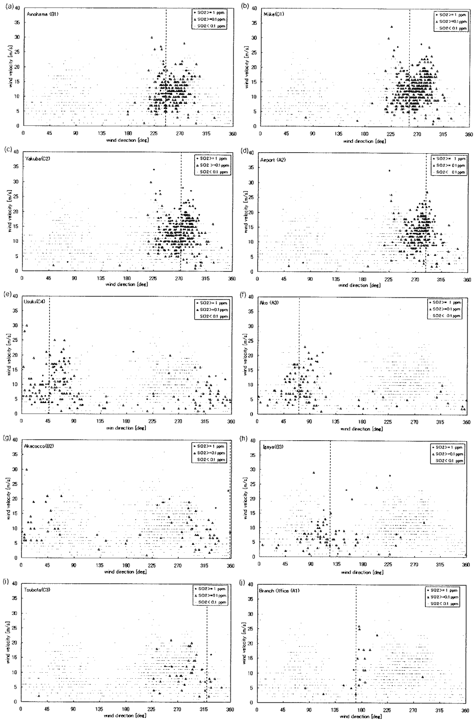
図5 高層風観測時に測定されたSO 2 濃度に対する八丈島925 hPa風の風向と風速の散佈図 (a) 逢の浜局 (B1), (b) 三池局 (C1), (c) 役場局 (C2), (d) 空港局 (A2), (e) 薄木局 (C4), (f) 阿古局 (A3), (g) アカッコ局 (B2), (h) 伊ヶ谷局 (B3), (i) 坪田局 (C3), (j) 支庁局 (A1). ● : SO 2 ≥ 1 ppm, △ : 0.1 ppm ≤ SO 2 < 1 ppm, × : SO 2 < 0.1 ppm 各局からの火口の方向を点線で示す。
