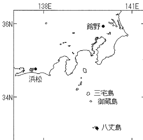
図1 三宅島及び周辺の高層風観測点(●)とwebカメラが設置された御蔵島の位置
