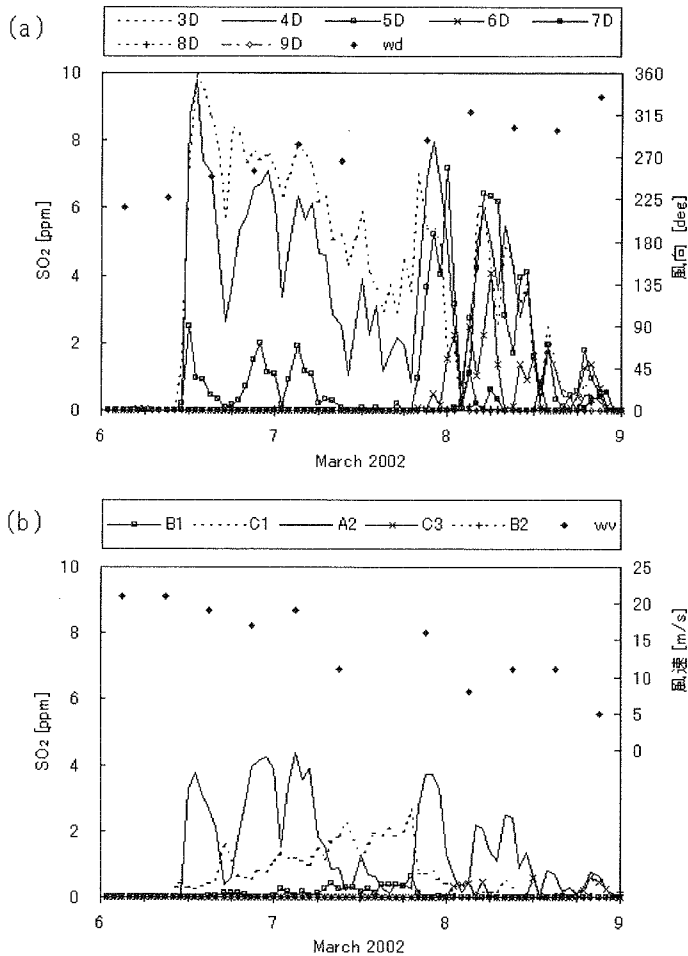
図8 2002年3月6～8日のSO 2 濃度の時系列変化と八丈島925hPa風(a)山腹局,(b)山麓局
